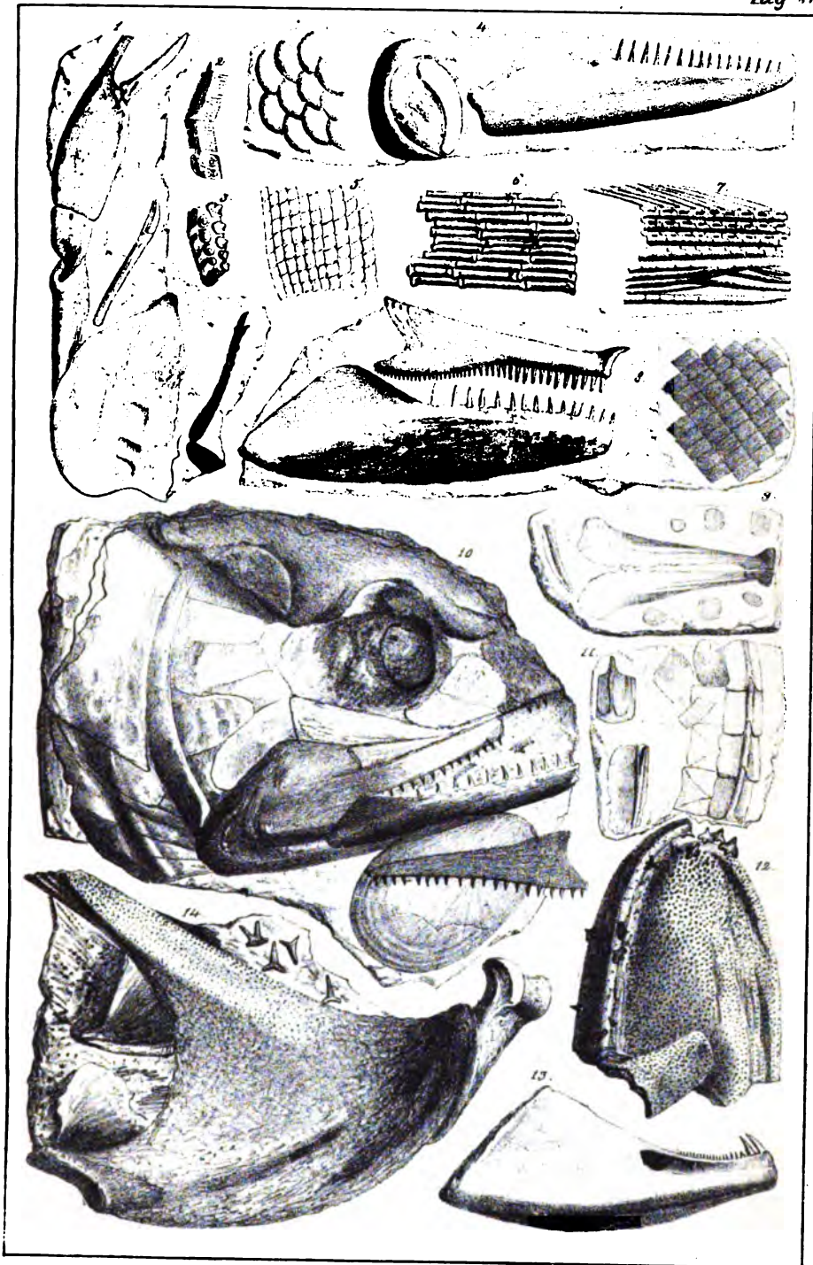
Quensbedt, Jura.
